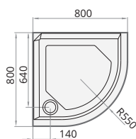
CL RO 80 R 550
